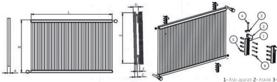
1- Askı aparatı 2- Askılık 3- Askı kapağı 4- Askılık vidası 5- Döbel
