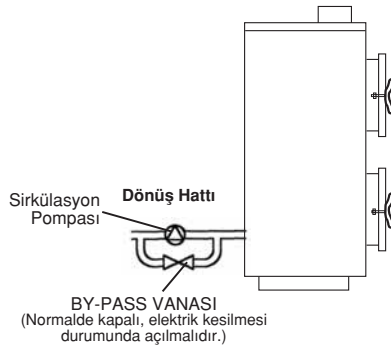
Şekil 2 : By-Pass Hattının Yapılması
