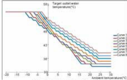
Heating Mode için yüksek sıcaklık eğrileri
